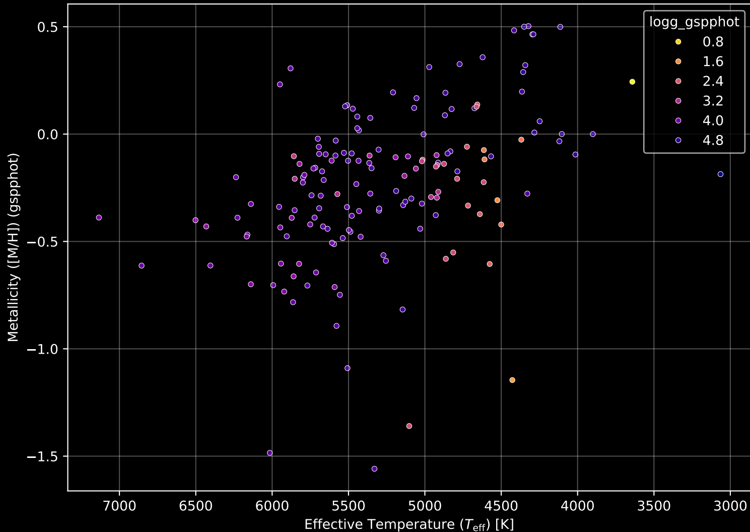
APOGEE DR17 Field: [038+48_MGA] Stellar Population Parameters (n= 159)
